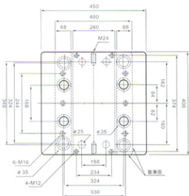
平面圖
