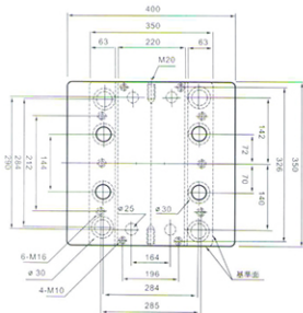
平面圖
