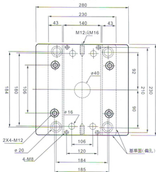
平面圖
