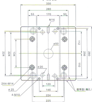
平面图
