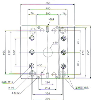
平面圖
