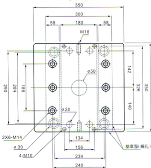
平面圖
