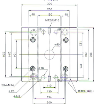
平面圖
