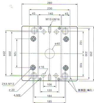
平面圖
