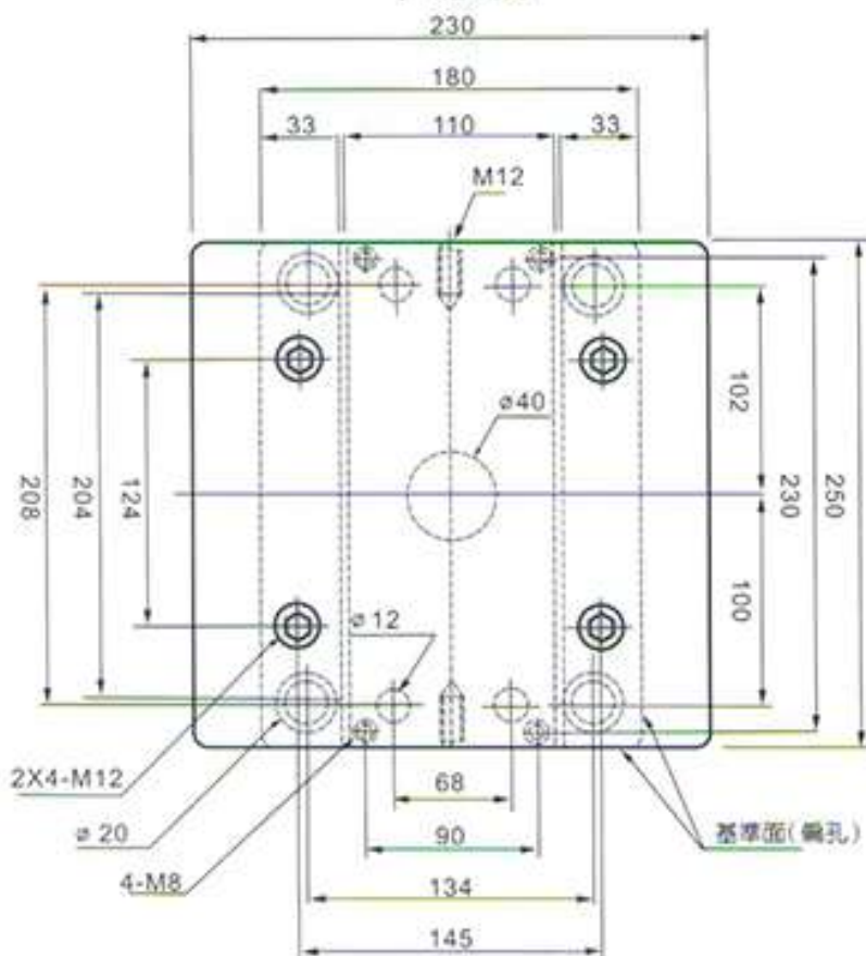
平面圖
