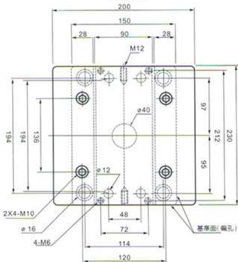
平面圖
