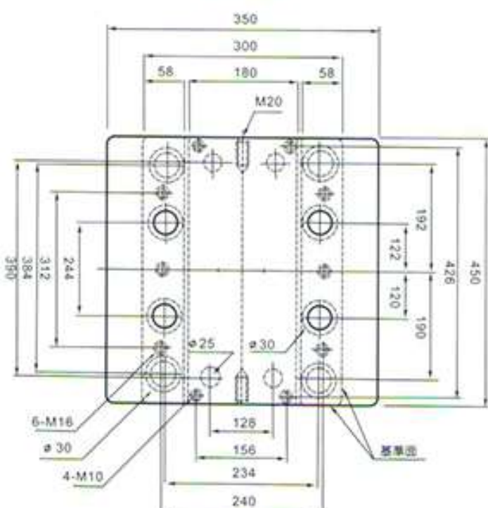
平面圖
