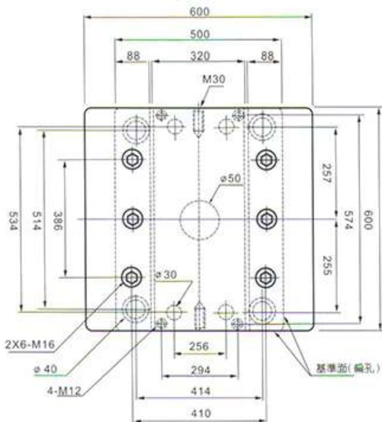
平面圖
