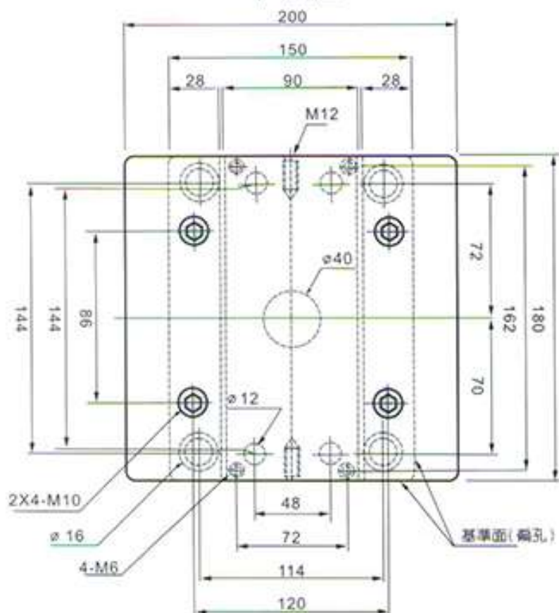
平面圖
