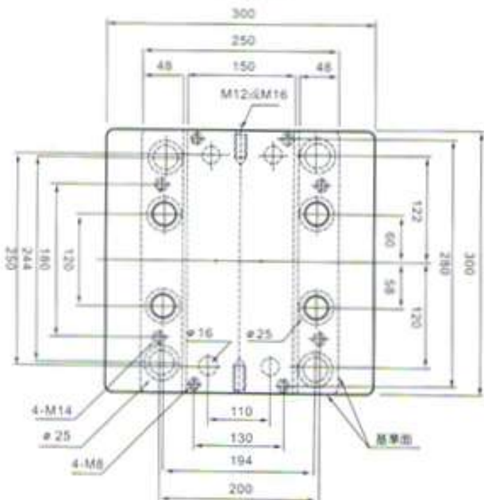
平面圖
