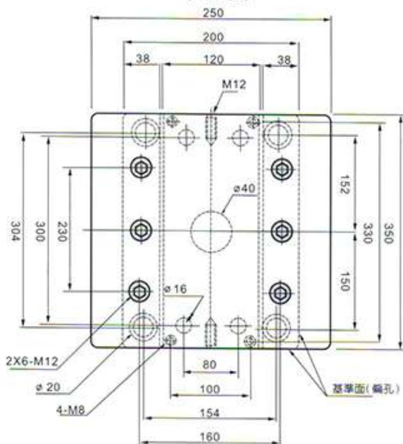
平面圖
