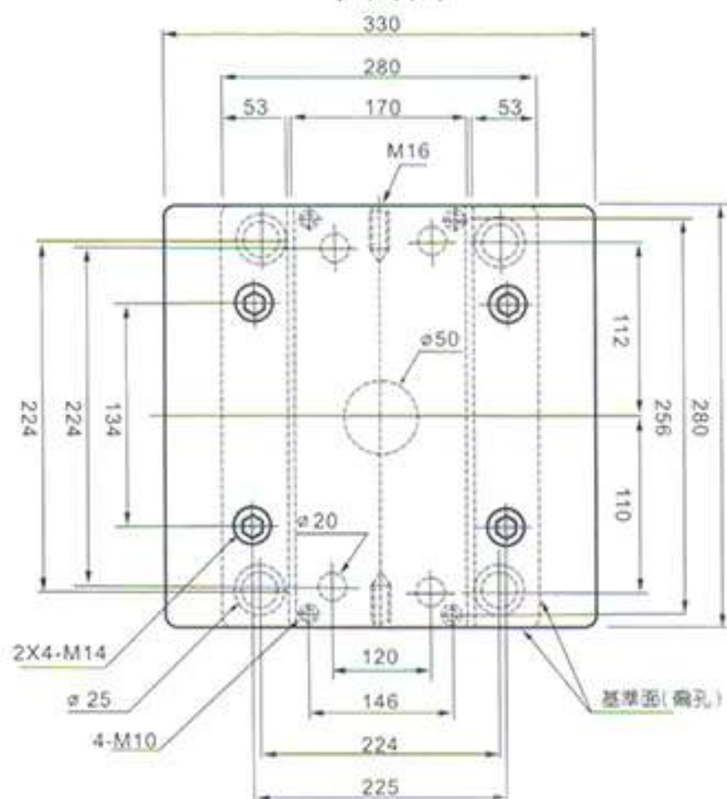
平面圖
