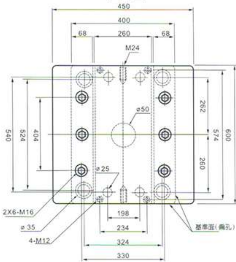
平面圖
