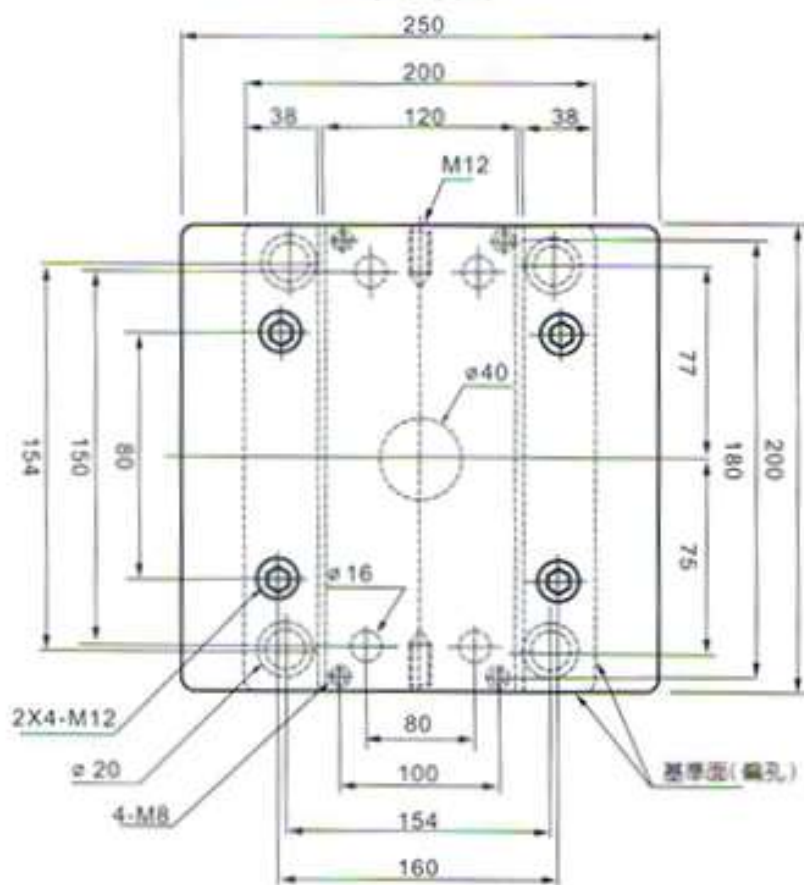
平面圖
