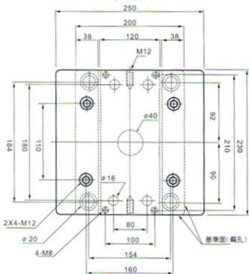
平面圖
