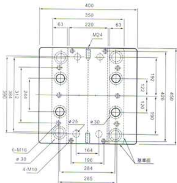
平面圖
