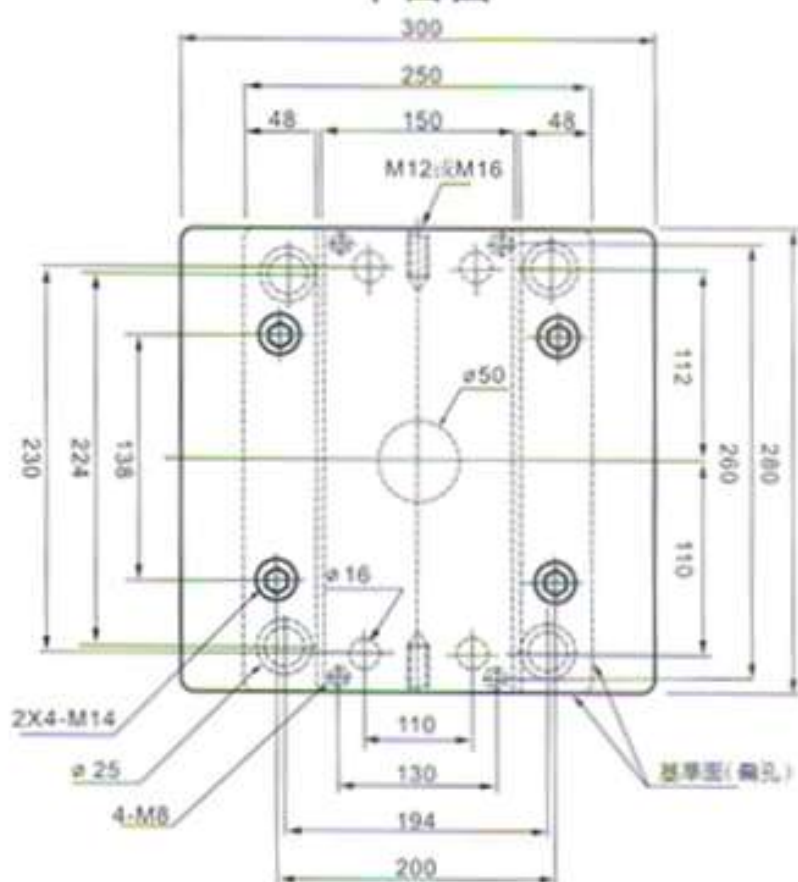
平面圖
