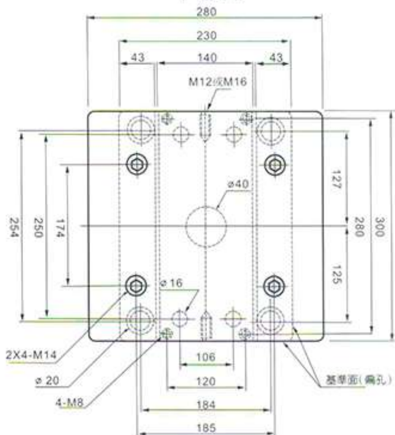
平面圖
