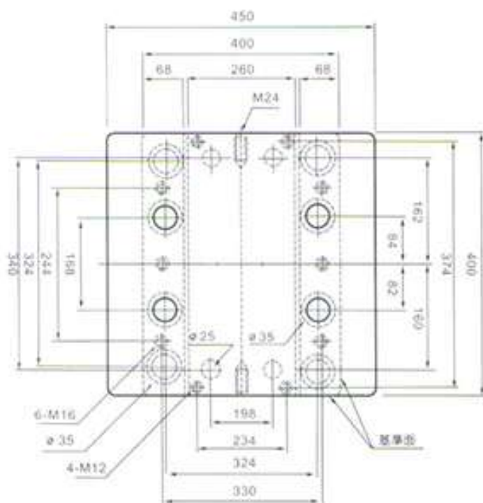
平面圖
