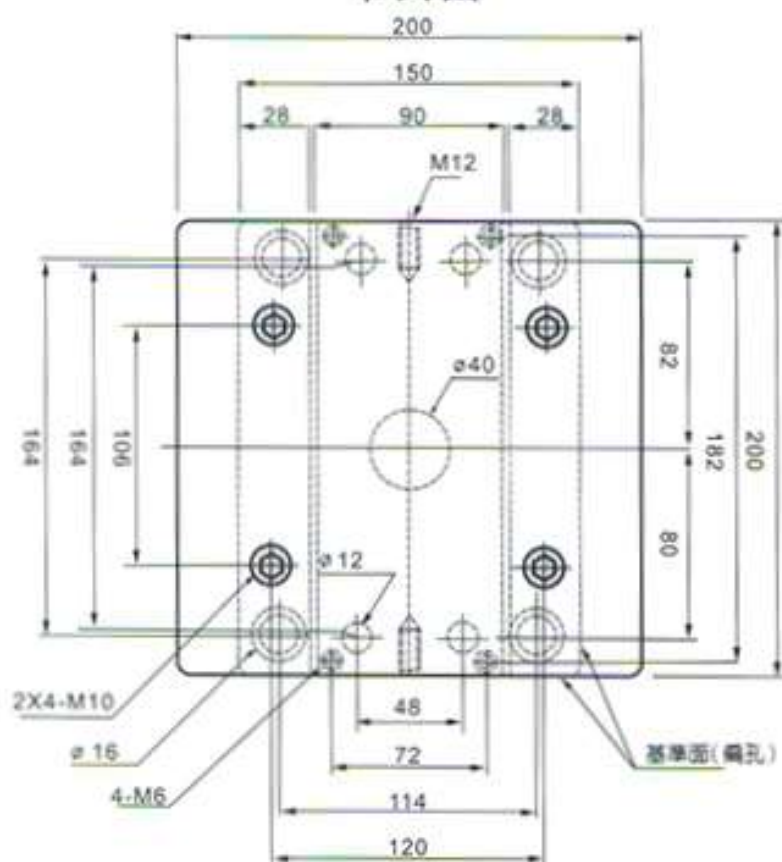
平面圖
