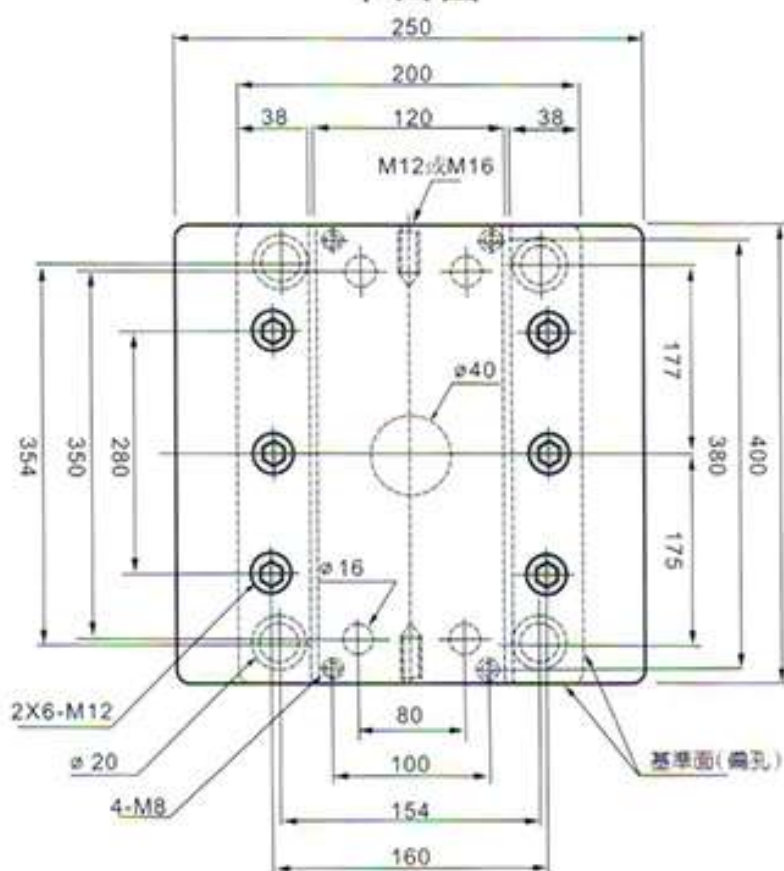
平面圖
