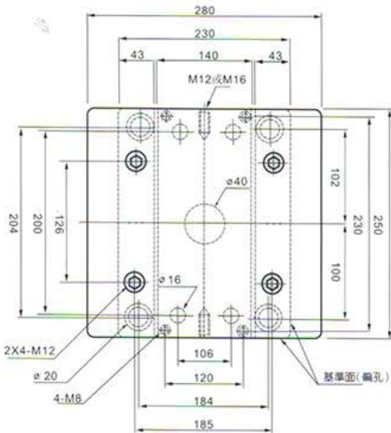
平面圖
