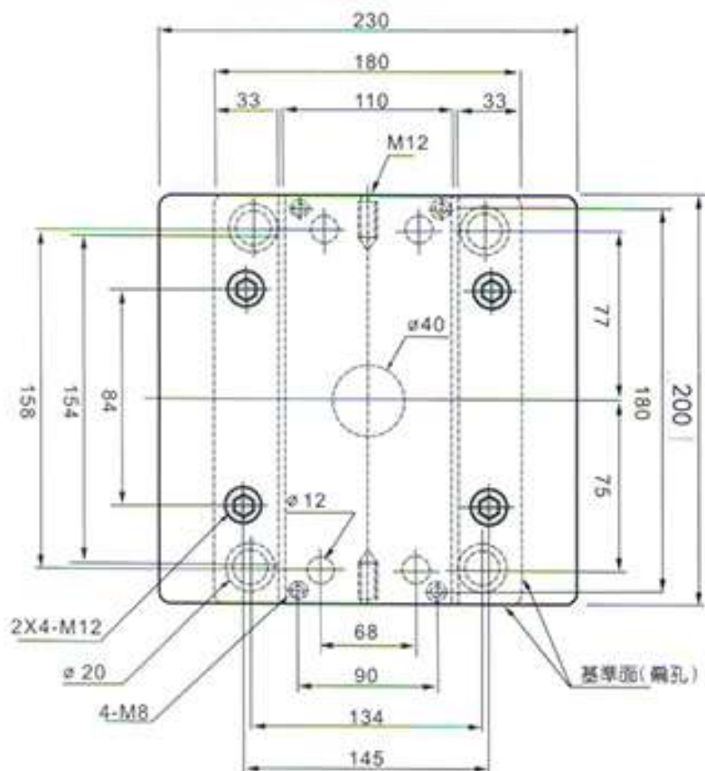
平面圖
