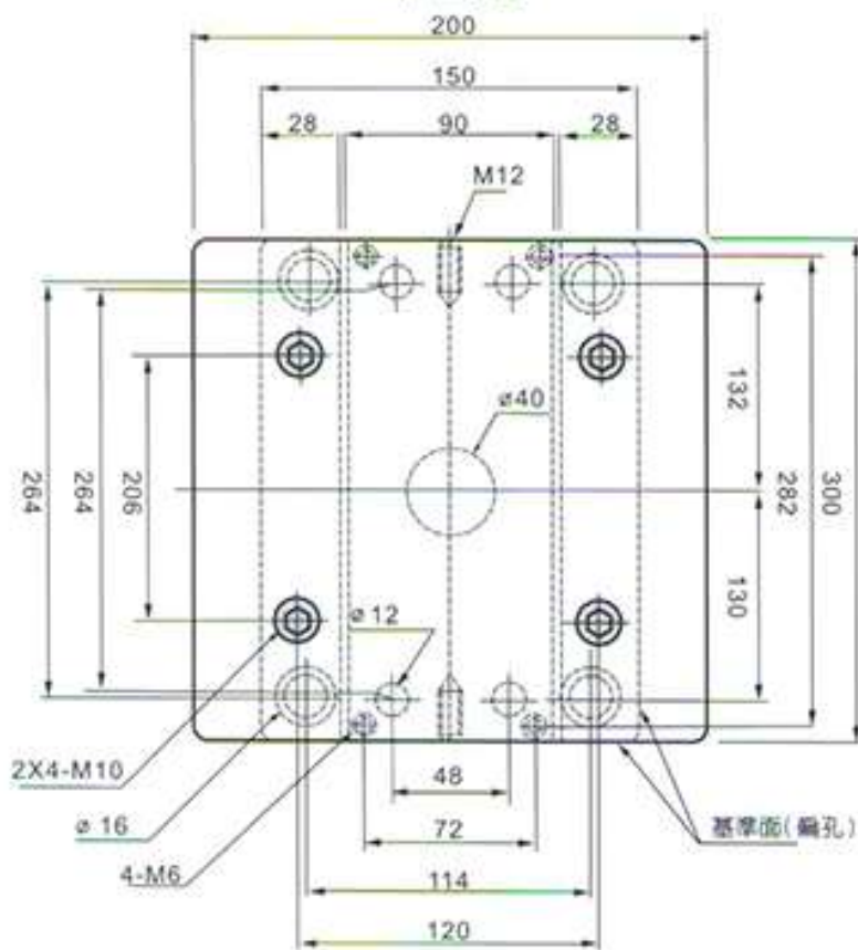
平面圖
