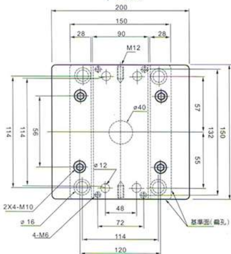
平面圖
