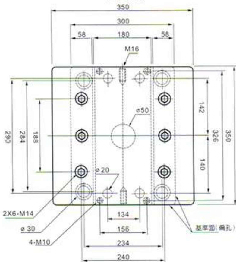
平面圖
