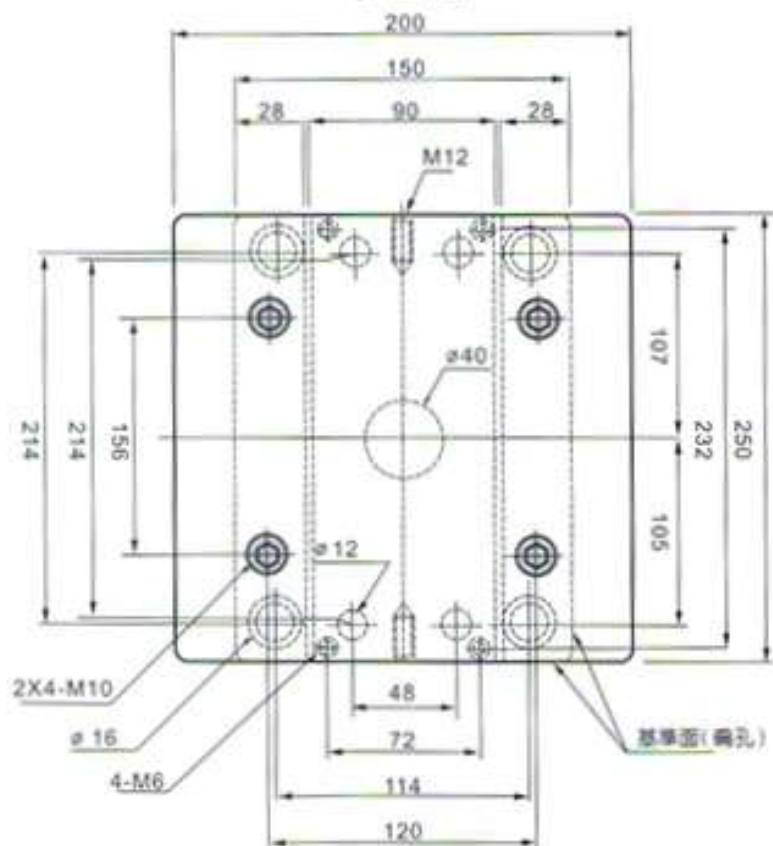
平面圖
