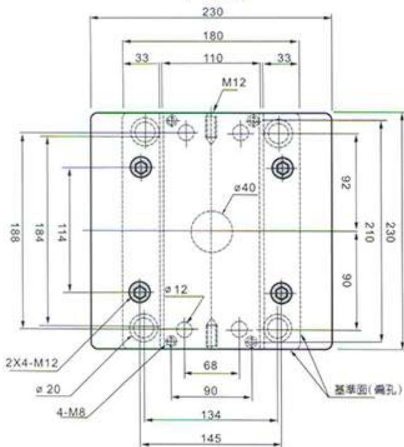
平面圖
