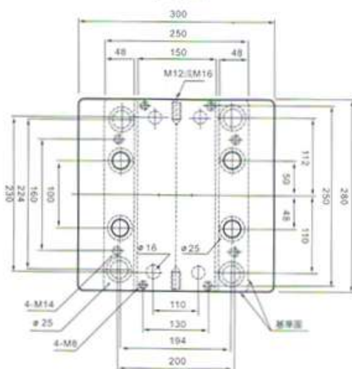
平面圖
