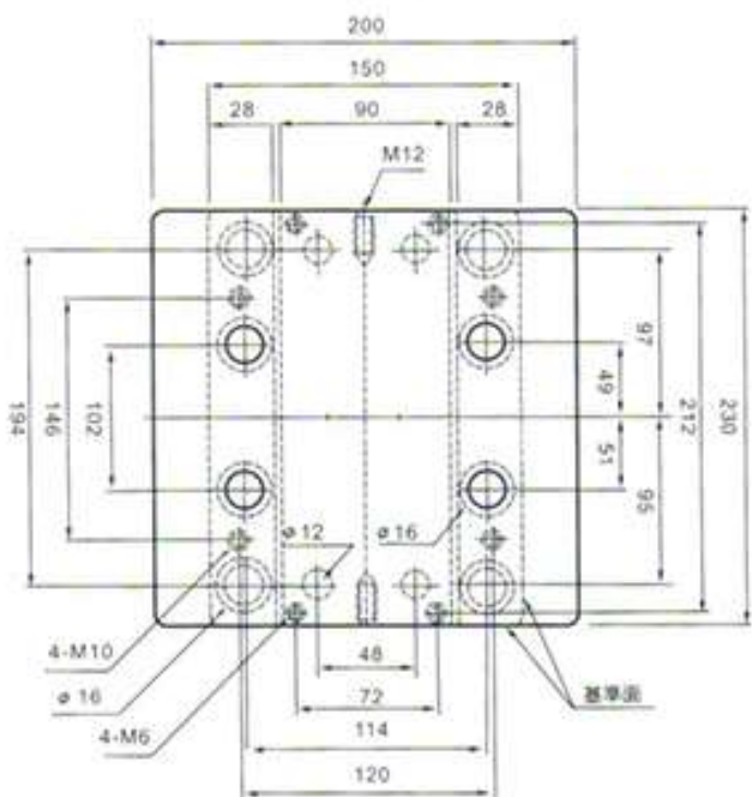
平面圖
