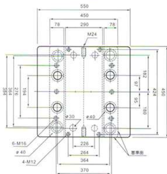
平面圖
