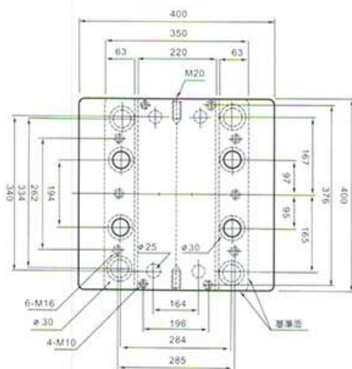
平面圖
