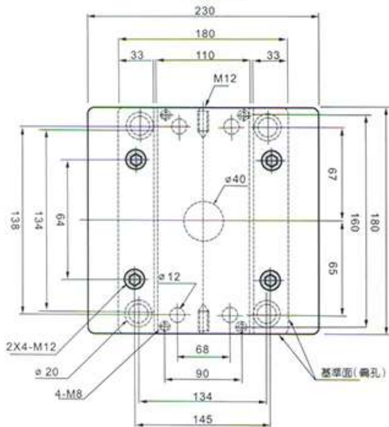
平面圖
