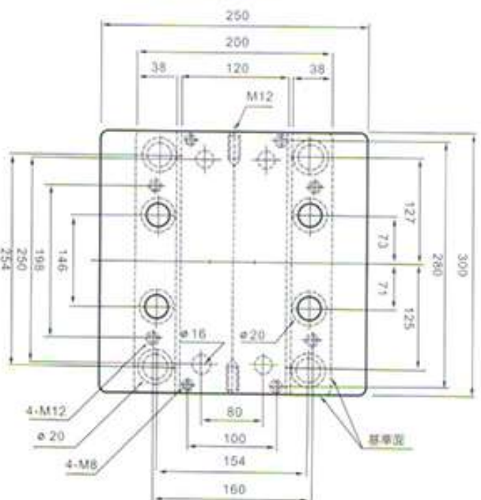
平面圖
